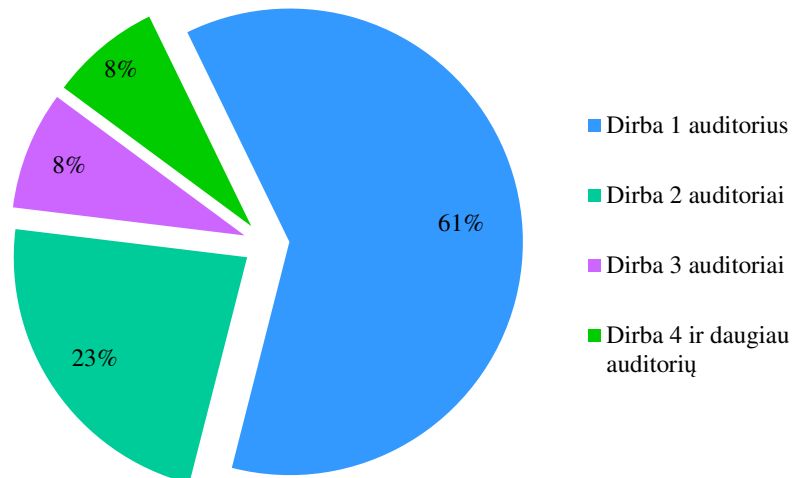
13 pav. Audito įmonių pasiskirstymas pagal jose dirbančių auditorių skaičių 2012 metais
