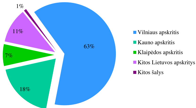
4 pav. Auditorių pasiskirstymas pagal gyvenamąją vietą Lietuvos apskrityse 2012 metais
