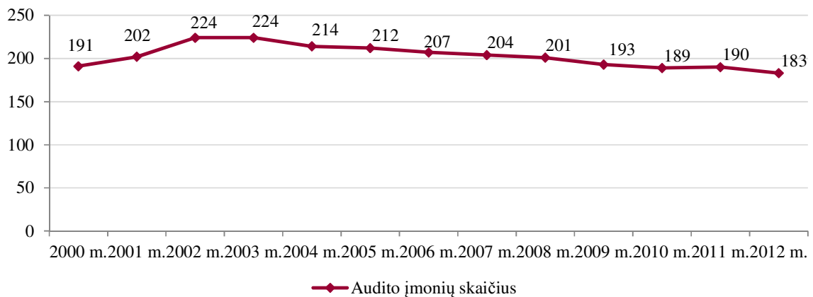
10 pav. Audito įmonių skaičiaus pokytis 2000–2012 metais
