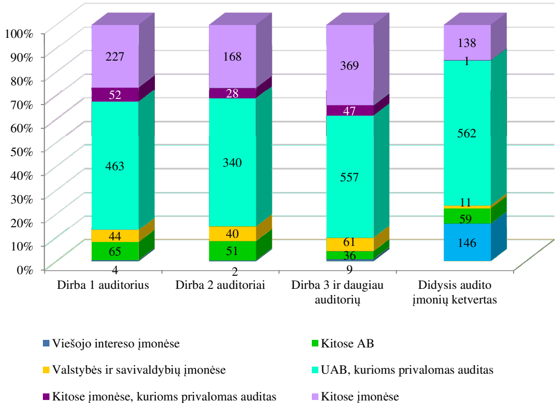
17 pav. Atliktų metinių auditų skaičius pagal audito įmonėse dirbančių auditorių skaičių ir audituotų įmonių formas 2012 metais
