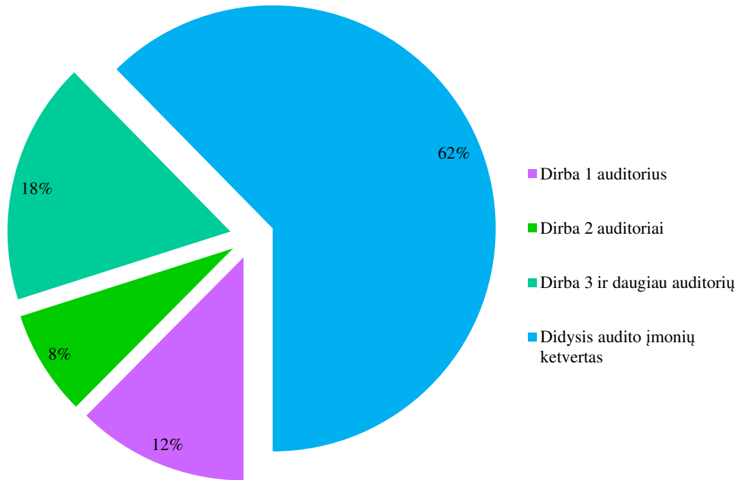
19 pav. Audito įmonių pajamų pasiskirstymas pagal jose dirbančių auditorių skaičių 2012 metais
