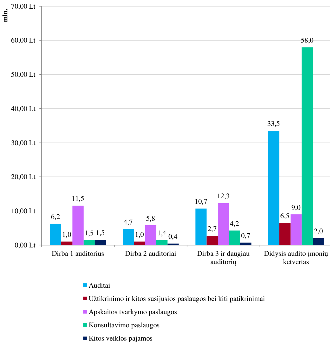
20 pav. Audito įmonių pajamų pasiskirstymas pagal veiklos rūšis ir audito įmonėse dirbančių auditorių skaičių 2012 metais
