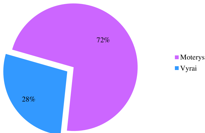
6 pav. Auditorių vyrų ir moterų, užimančių audito įmonės vadovo pareigas, pasiskirstymas 2012 metais
